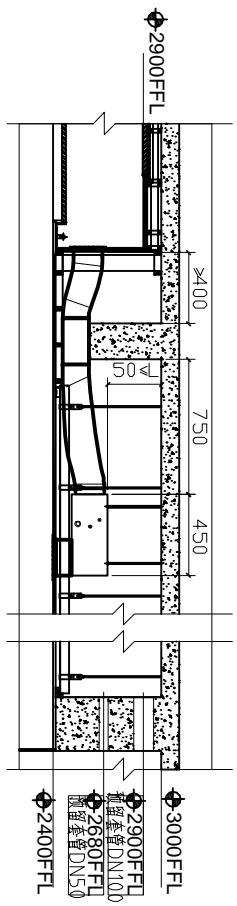
客卧一空调室内机安装剖面图 1:40
